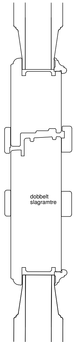
horisontalsnitt
