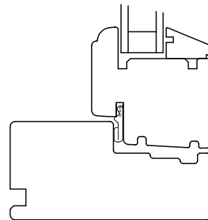
horizontalsnitt
