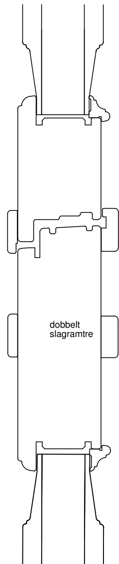
horizontalsnitt
