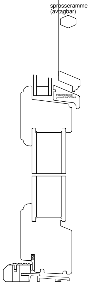
HC terskel vertikalsnitt
